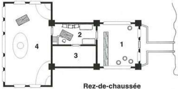
Rez-de-chaussée
